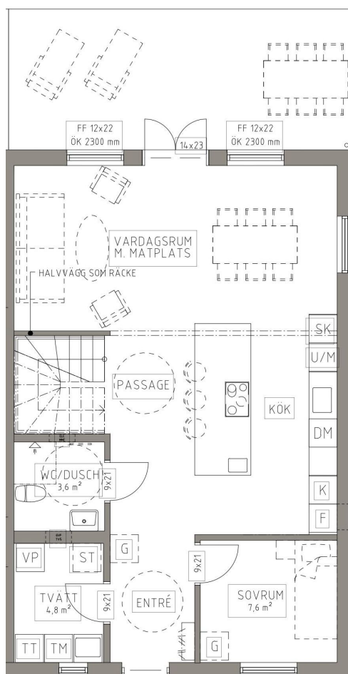
ENTRÉPLAN
